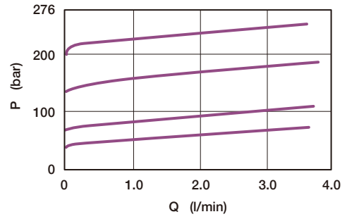
▶ 압력 차 vs. 유량 (범위 A)
